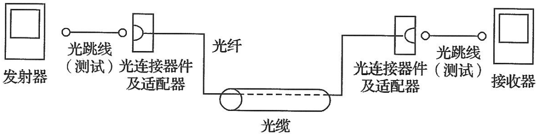
图 C.0.3 光纤链路测试连接(单芯)
