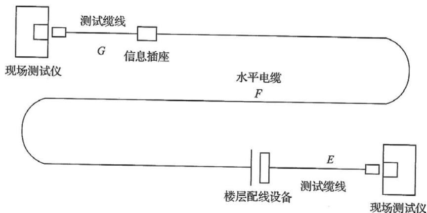
图 B.0.1-1 基本链路方式
