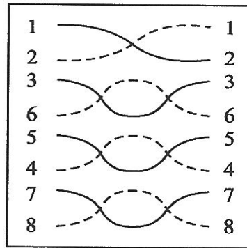
(b) 反向线对
