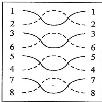
(a) 正确连接
