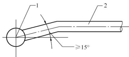
图 3.4.6 排水横管的水平连接
